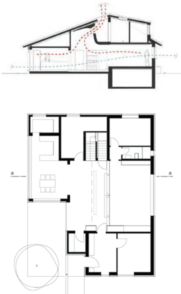
Schnitt und Grundriss des umgebauten Hauses
